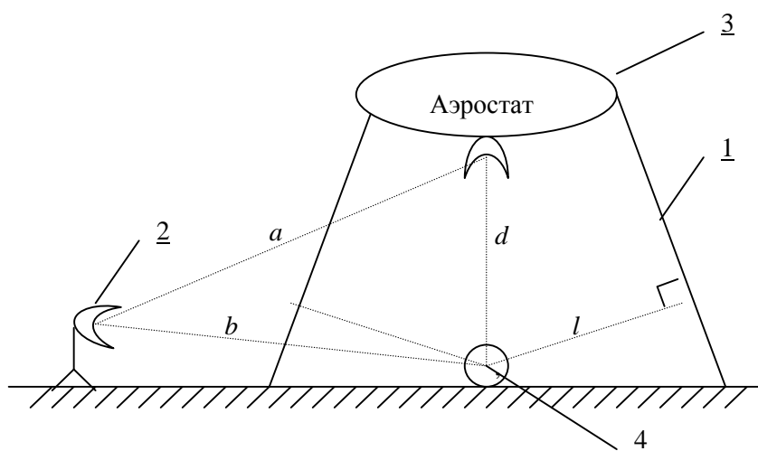
Рисунок 1. Реализация способа защиты радиолокационных станций от противорадиолокационных ракет на основе пассивных источников излучения.
