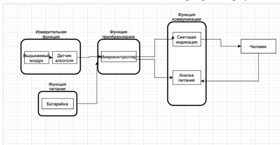
Рисунок 1. Функциональная структура прибора
