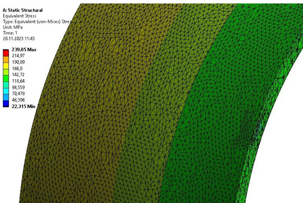
Рисунок 3 - Напряжение на ремонтной муфте.
