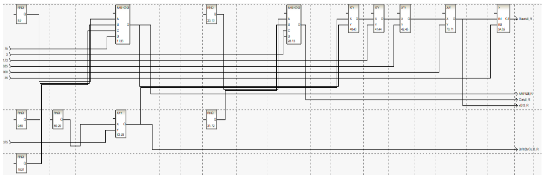
Рисунок 2 – Алгоритм управления передачи данных с анализатора сети на графическом языке программирования FBD
