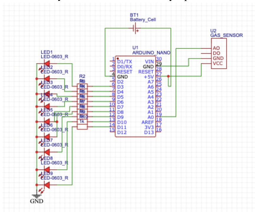
Рисунок 3. Схема подключения
