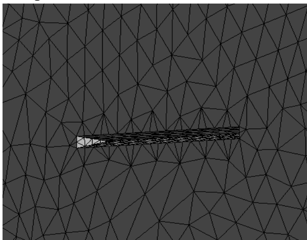
Рисунок 1 – расчетная сетка элемента нефтепровода с повреждением глубиной 3 мм.
