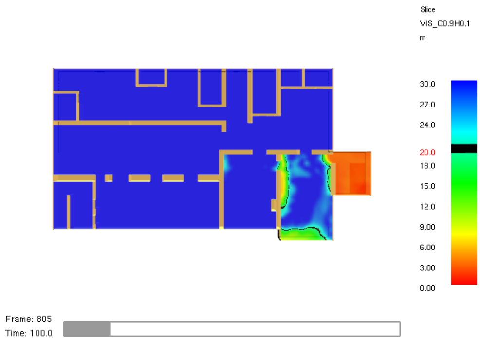
Рисунок 2 – Дальность видимости на 100 секунде пожара
