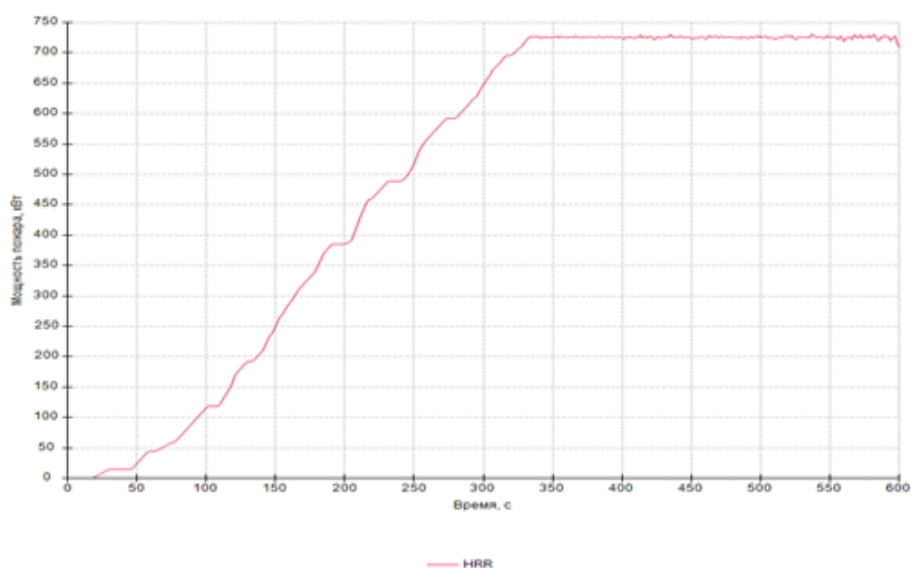
Рисунок 5 – График мощности пожара
