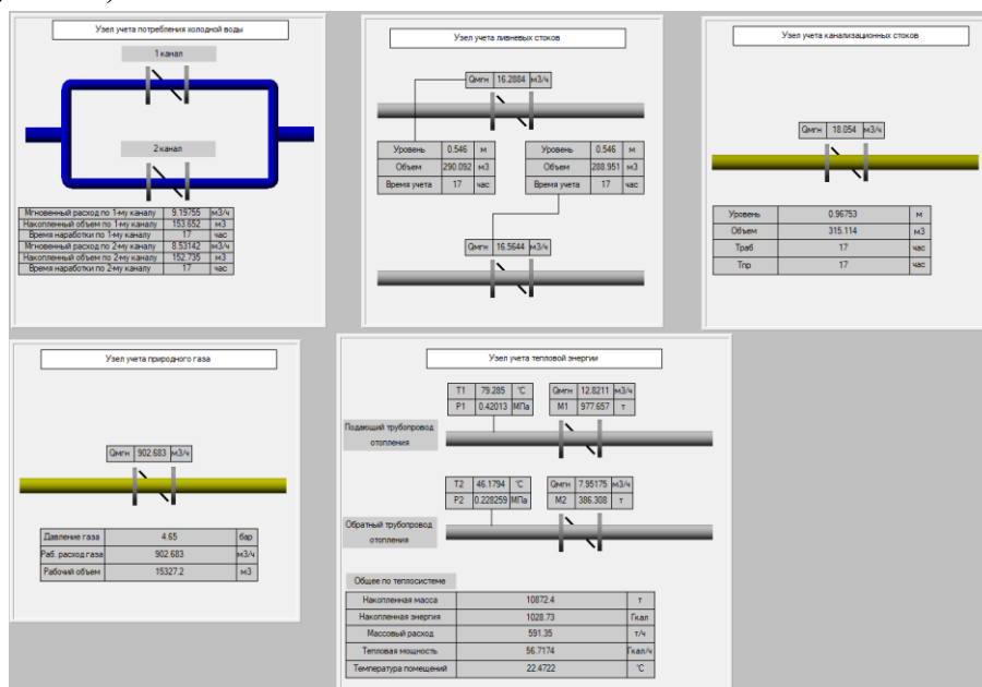
Рисунок 1 – Мнемосхема узлов учета
