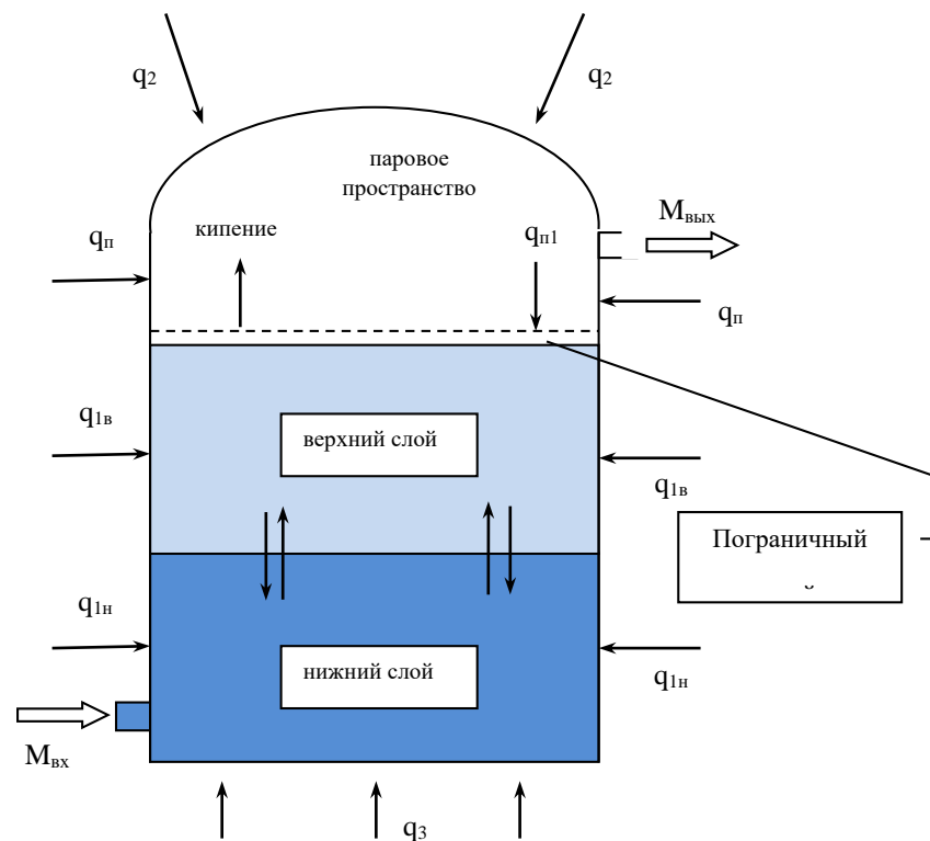
Рис. 1. Стратификация слоев при закачке продукта в резервуар q_{1н} – тепловой поток через стенку к нижнему слою; q_{1в} – тепловой поток через стенку к верхнему слою; q_2 – тепловой поток через покрытие к парогазовой фазе; q_3 – тепловой поток через днище; q_{п} – тепловой поток через стенку к парогазовой фазе; q_{п1} – тепловой поток от парогазовой фазы к жидкости; M_{вх} – скорость закачки продукта, кг/с; M_{вых} – скорость отбора паров СПГ из резервуара, кг/с
