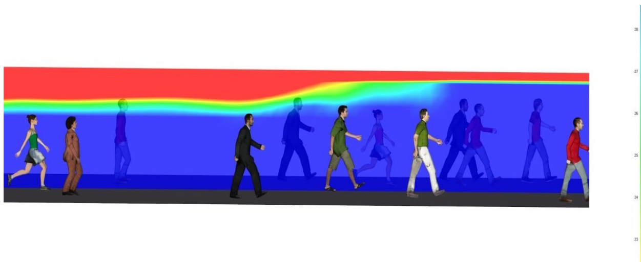
Рисунок 2 – Визуализация полей опасных факторов пожара совместно с эвакуацией людей
