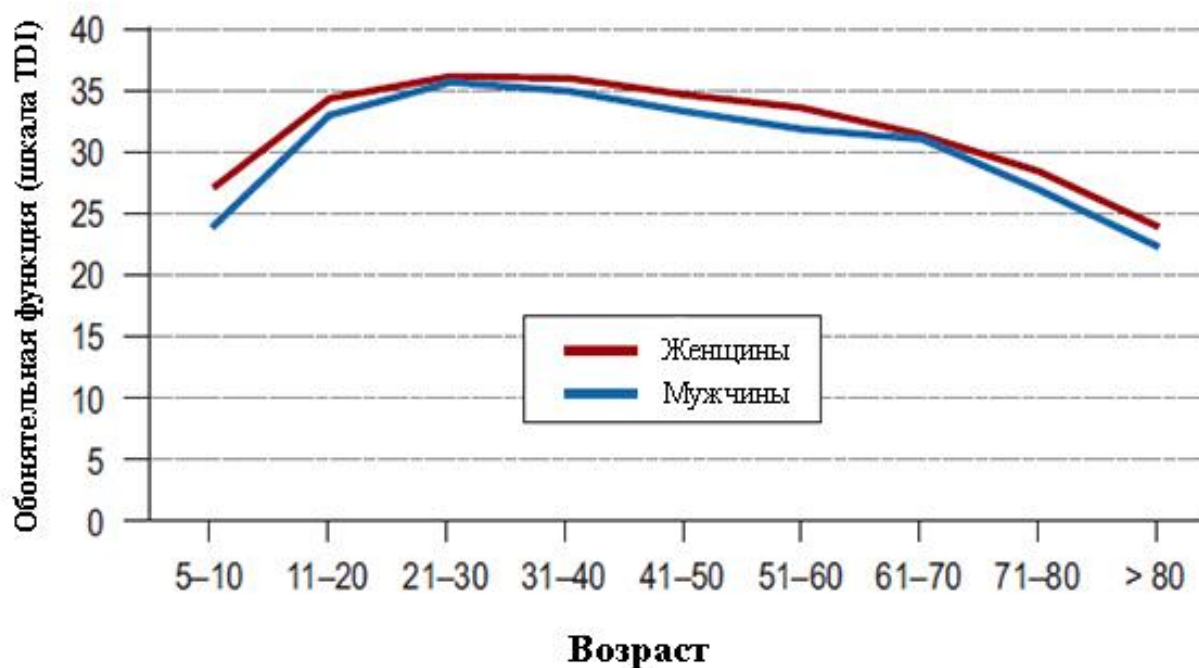
Рисунок 1. Возрастное изменение обонятельной функции у субъективно нормосмичных лиц ( n = 3355 ), стратифицированных по полу (модифицировано из [5]).
