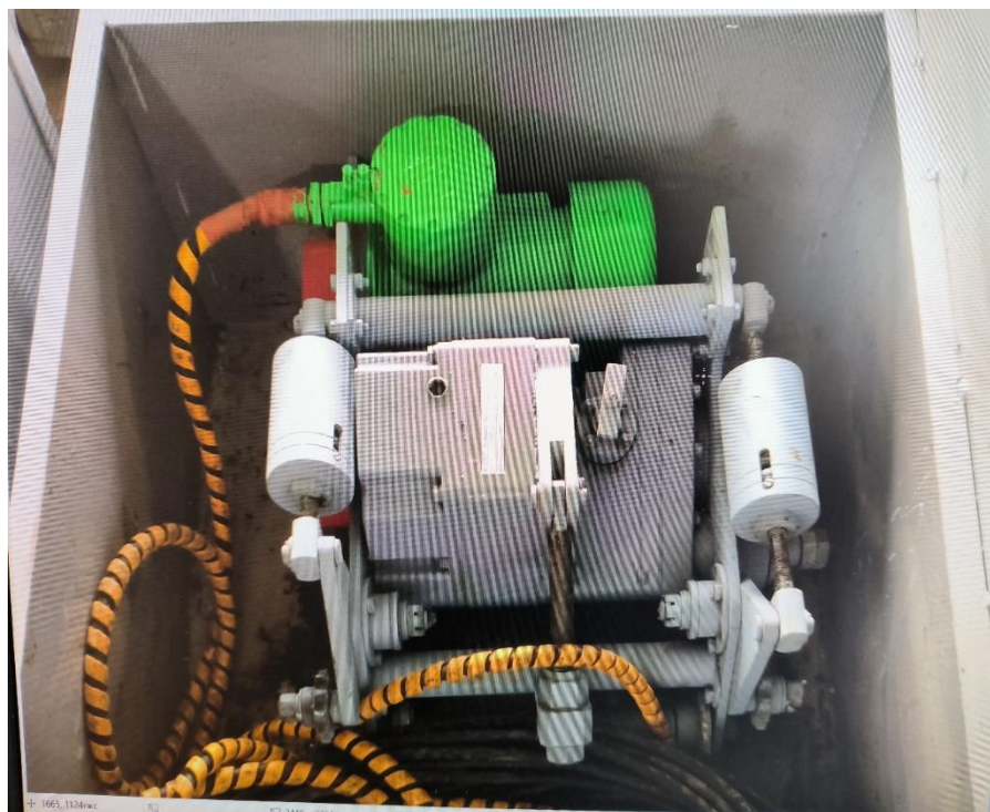
Рис.1 - МРТ "Волжанка-2"
