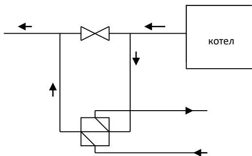
Рис. 2. Расчетная схема участка 1
