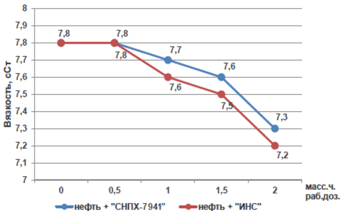
Рисунок 2. Зависимость вязкости нефти от концентрации ингибитора (164-ая скважина)
