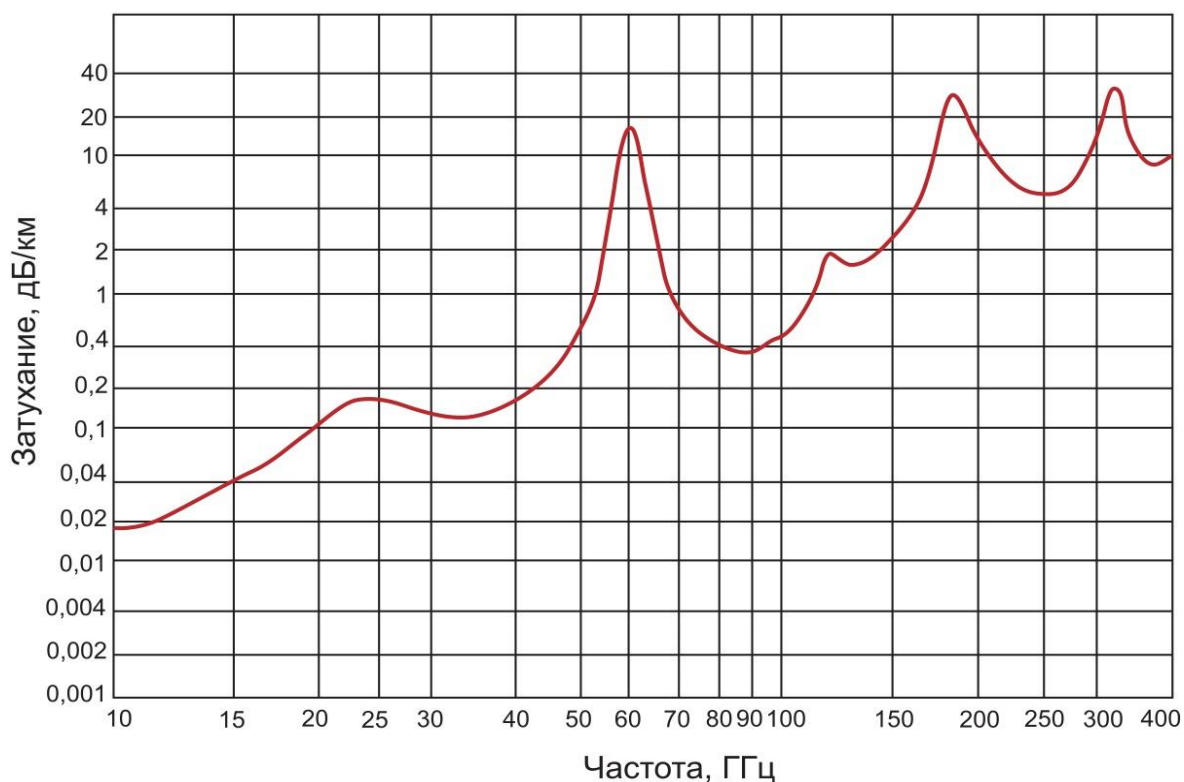
Рисунок 2. Зависимость коэффициента затухания от частоты
