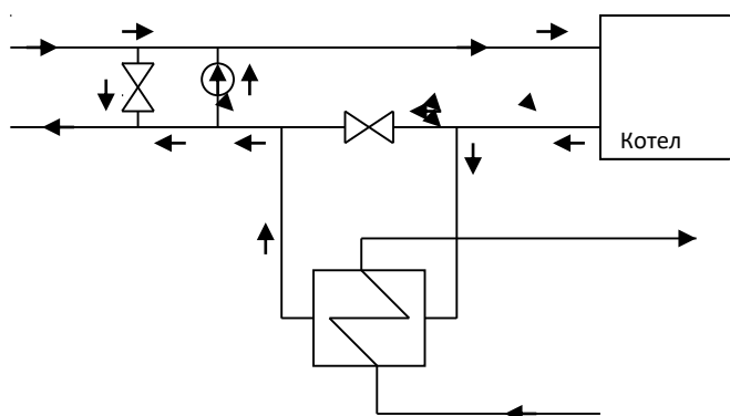
Рис. 1 Схема рециркуляции.
