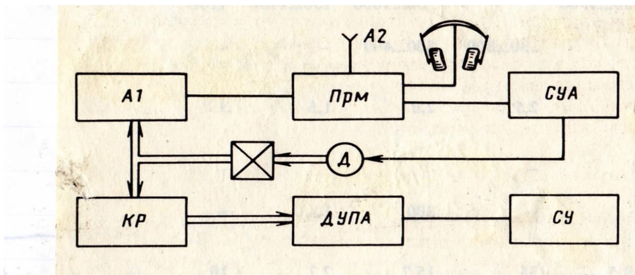
Рисунок 1. Состав радиокompаса
