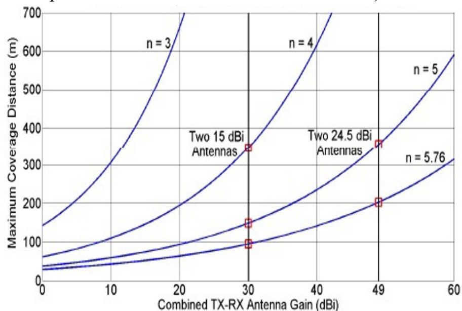
Рисунок 1. Зависимость расстояния покрытия от коэффициента усиления
