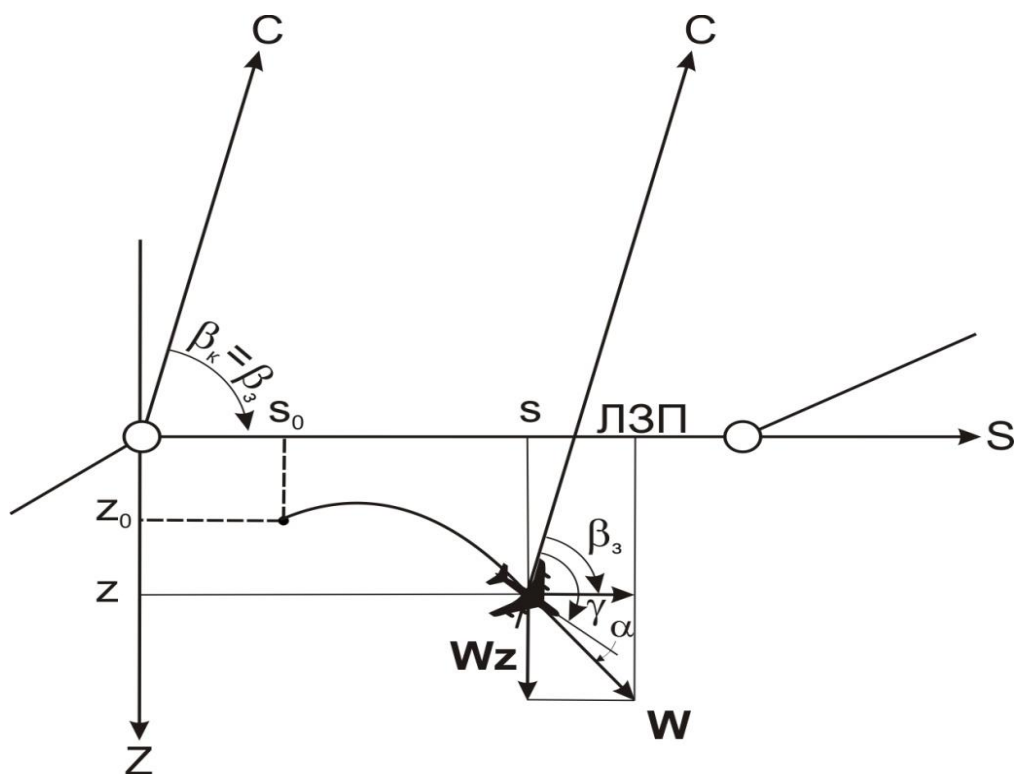
Рисунок 2 - Составляющие вектора путевой скорости
