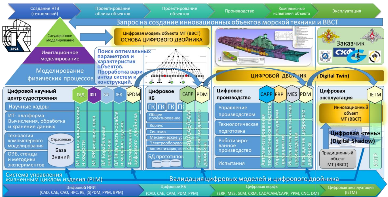
Рис. 4 Многоуровневая схема цифрового судостроения. [12]
