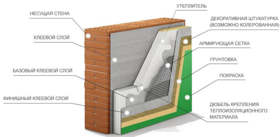
Рисунок 1 – Конструкция СФТК
