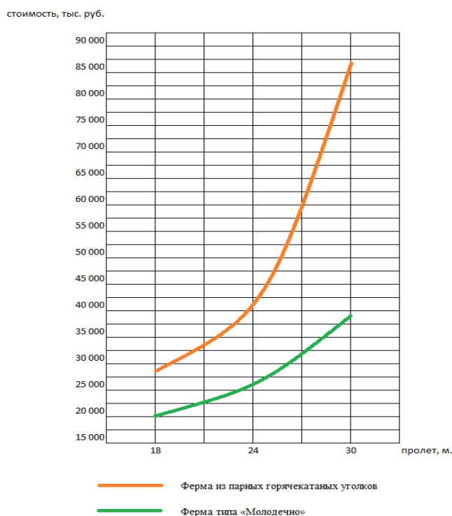
Рисунок 2. График зависимости стоимости монтажа от пролета конструкций покрытия
