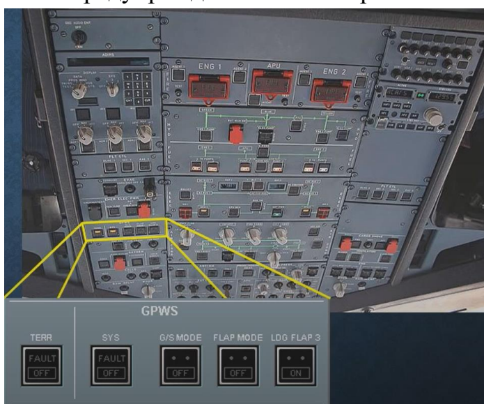
Рисунок 3. Расположение кнопок GPWS
