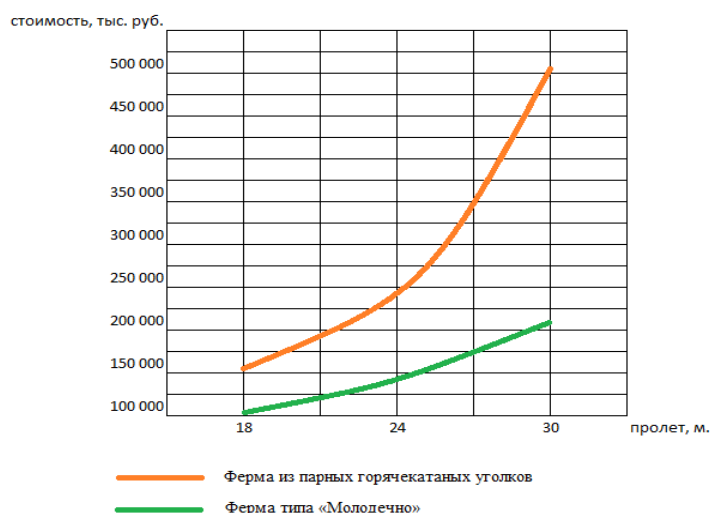
Рисунок 1. График зависимости стоимости изготовления от пролета конструкций покрытия
