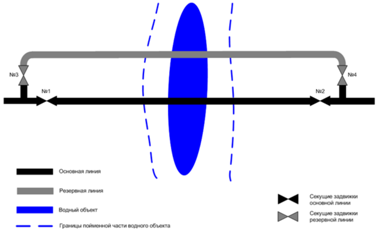
Рис.1 Схема монтажа резервной нитки
