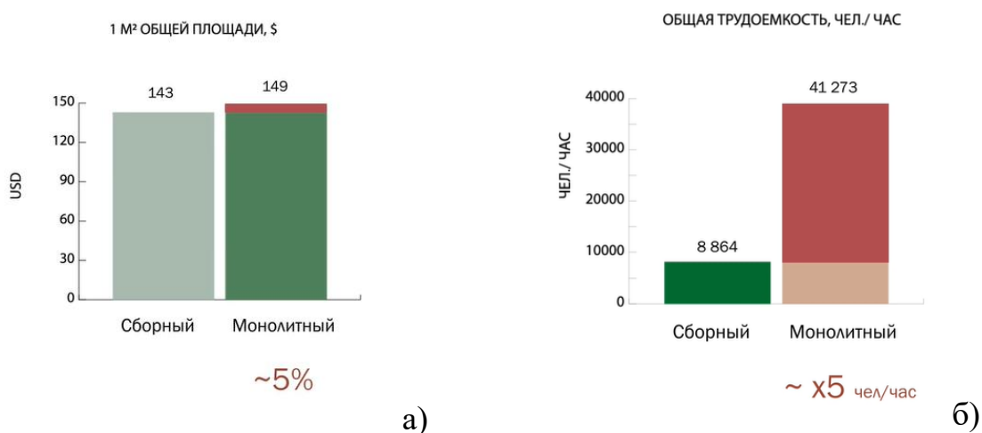
Рисунок 4. Результаты сравнения: а) в части стоимости объекта; б) в части общей трудоемкости.
