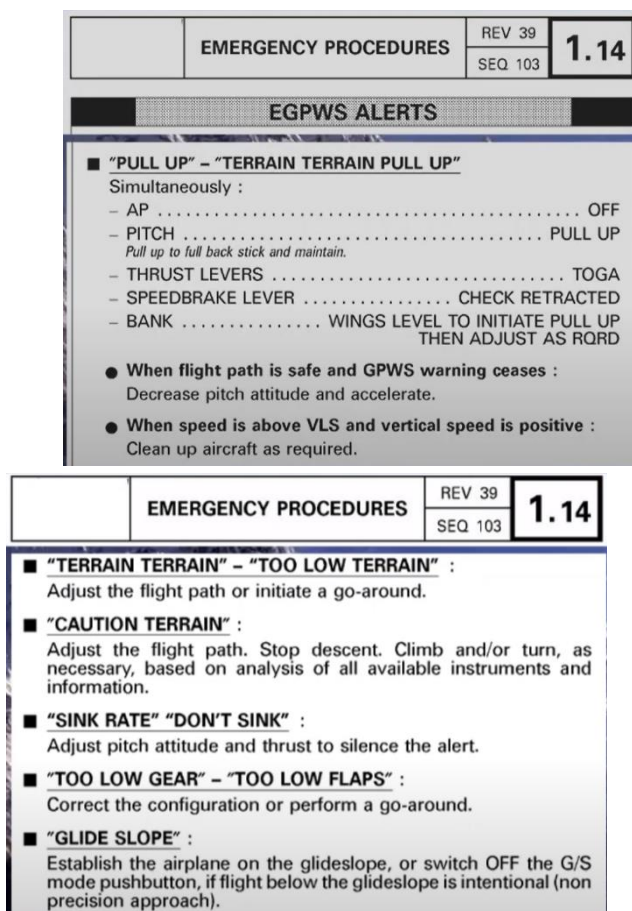
Рисунок 12. Режимы работы EGPWS
