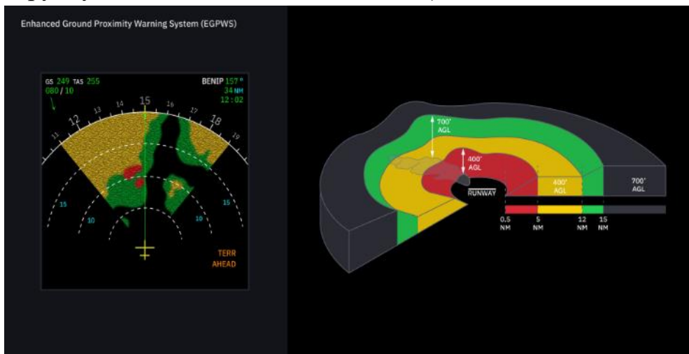
Рис.1 Отображения подстилающей земной поверхности на дисплее.
