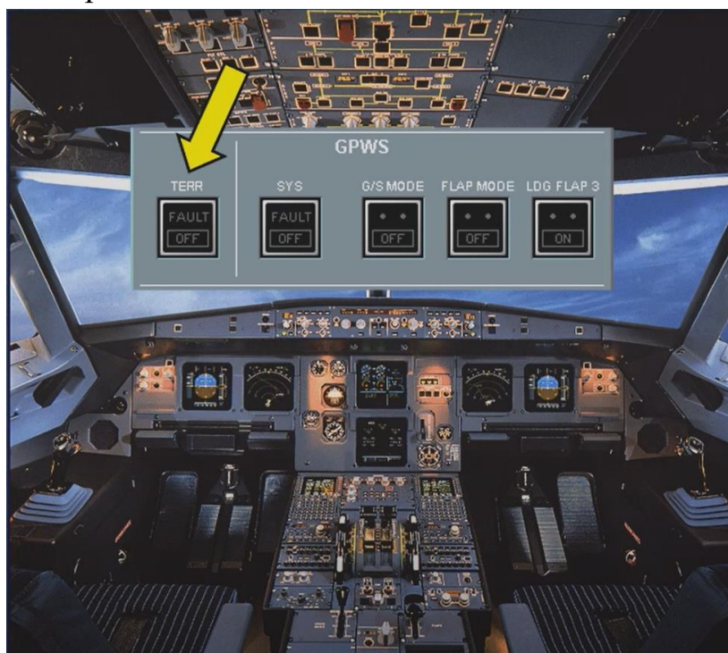
Рисунок 4. Вид кнопок GPWS
