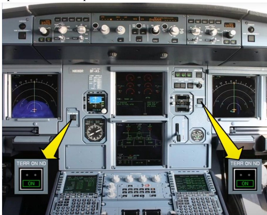
Рисунок 7. Расположение кнопок-индикаторов TERR ON ND
