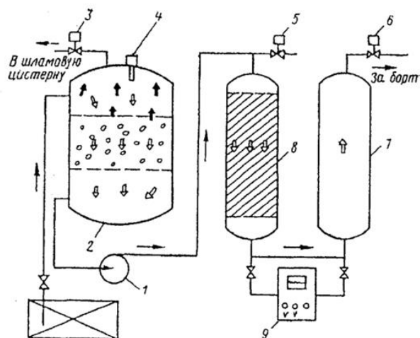
Рисунок 3. Схема очистки нефтеводной смеси в сепараторе системы «ПП МАТИК»
