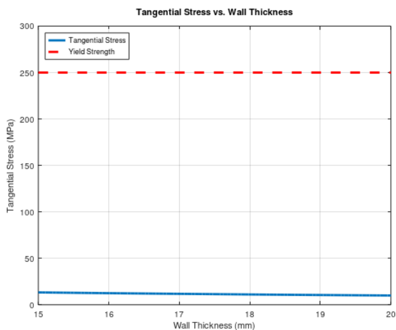
Рисунок 1 – Зависимость тангенциального напряжения от толщины стенки
