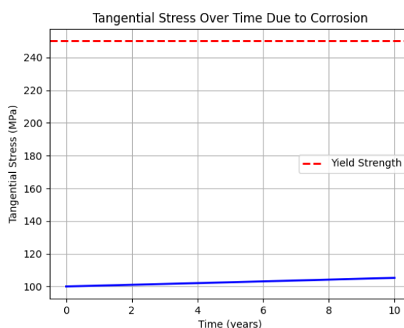
Рисунок 6 – Карта критических параметров тангенциальных напряжений
